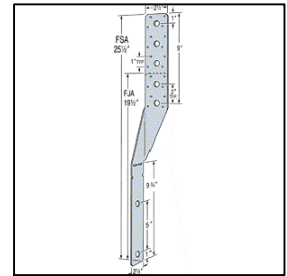
SK-4 (FJA)
